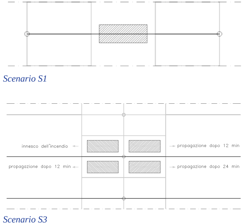
Illustrazione V.6-2: Schematizzazione degli scenari di incendio di progetto
